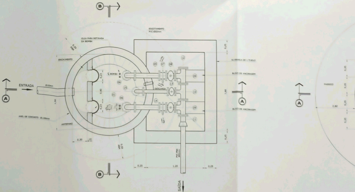
PLANTA NA COTA 695,500
