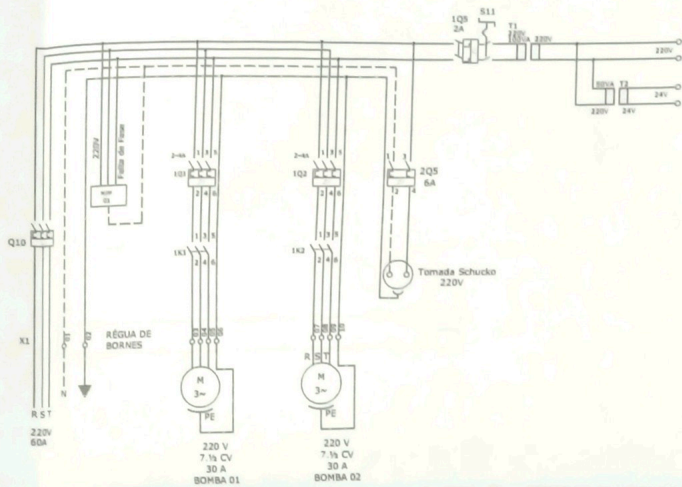
ESQUEMA TRIFILAR
