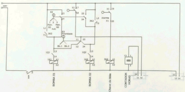
COMANDO ELÉTRICO
