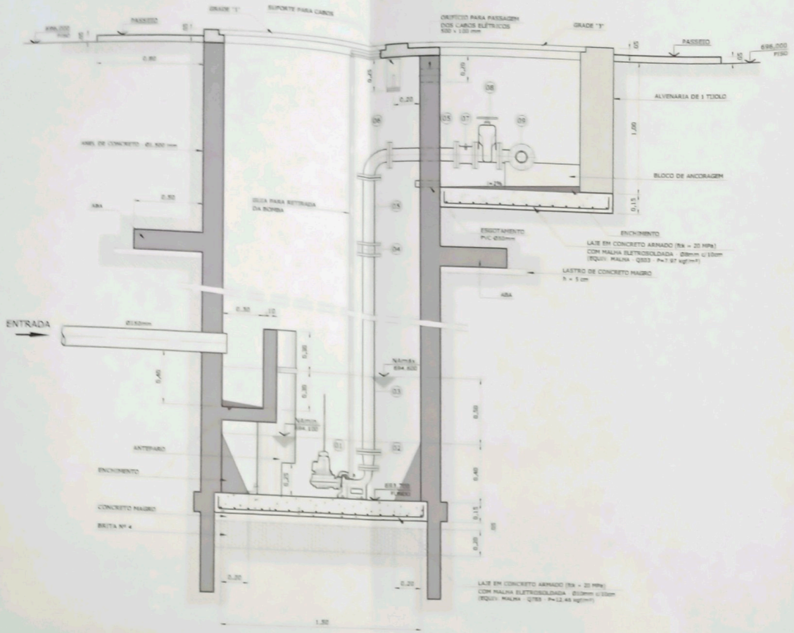
CORTE A-A ESC.: 1/20
