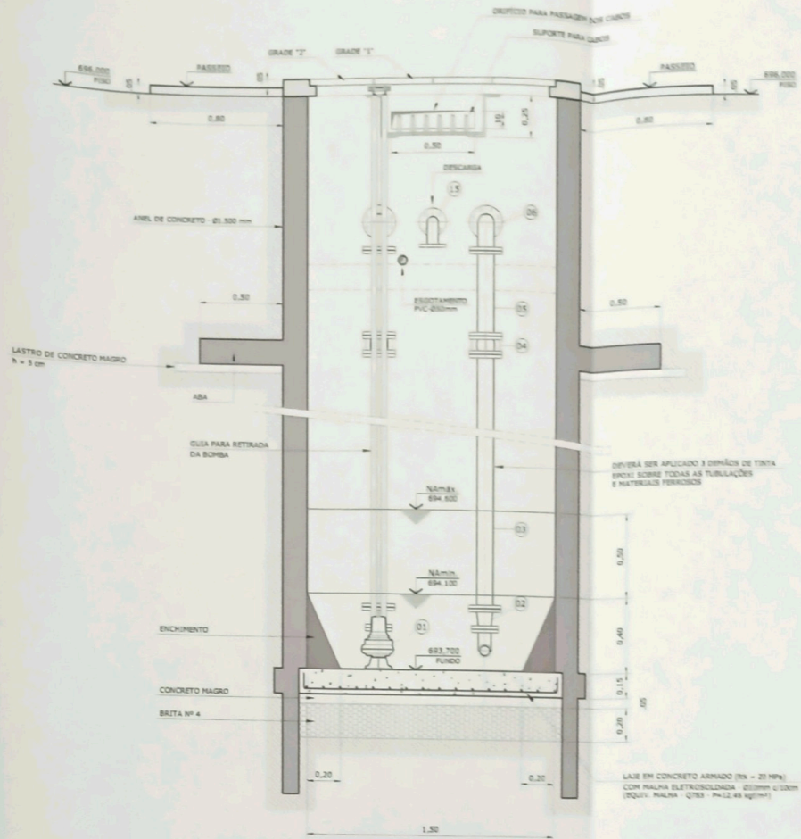
CORTE B-B
