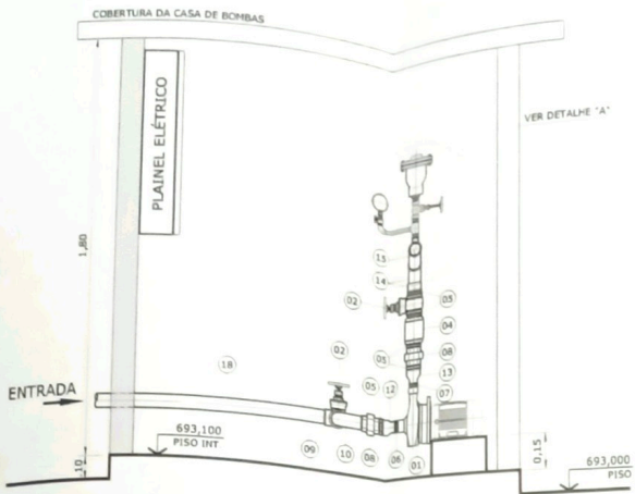
CORTE A-A
